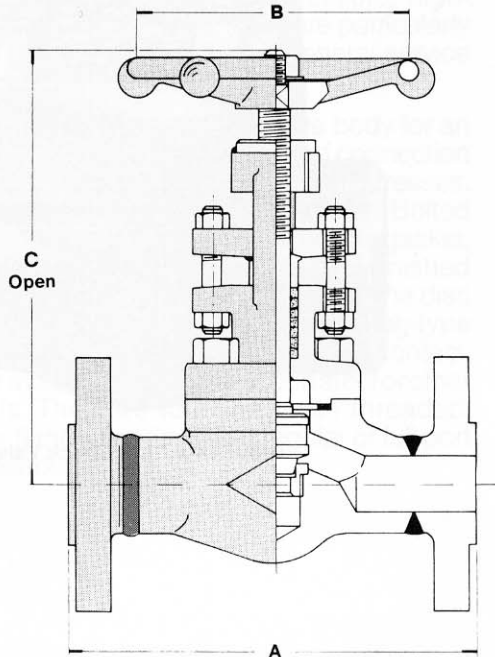
FB-3844XU-F
