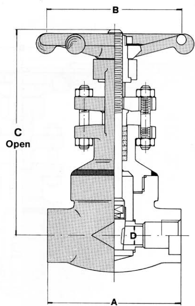
FW-3804XU-T FW-3804XU-W
