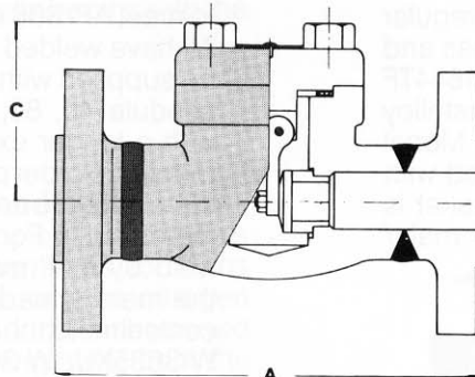
FB-3875XU-F SWING CHECK
