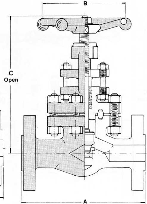
FB-3654XU-F Integral Flanges
